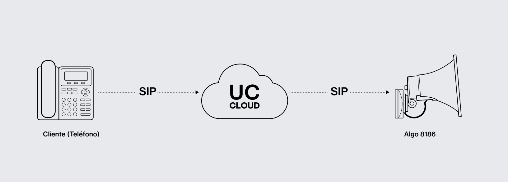
Diagrama de megafonía IP pura
